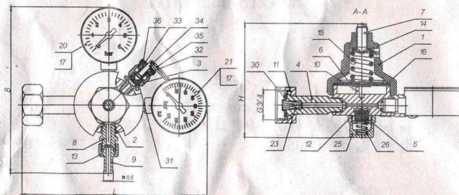
Рис.1 Редуктор баллонный углекислотный одноступенчатый.
